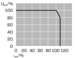
Ausgangskennlinie Output characteristic Puissance caractéristique
